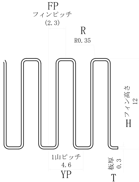
A部詳細(5倍)
